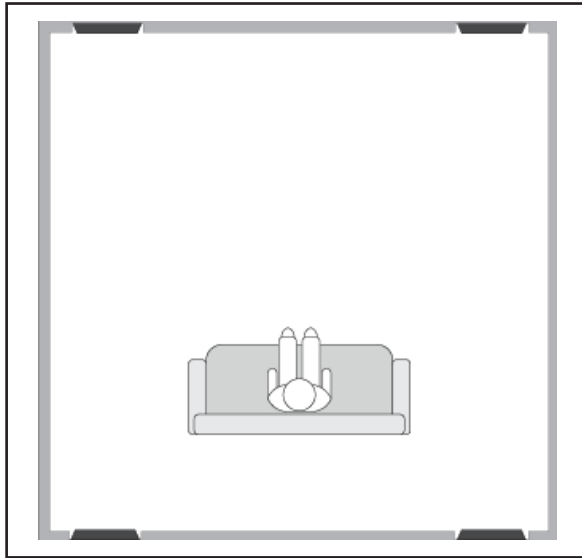
Rys. 1c Zalecane rozmieszczenie czterech subwooferów.
